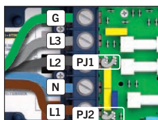
Monophasé avec un seul neutre
