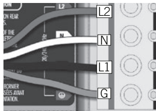
240 V (4 wires)
